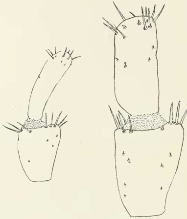
Fig. 3. Apis florea F. ♀. 3. und 4. Glied des rechten Läbials palpus von innen (vorn).
